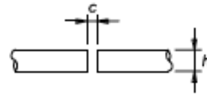
3) Bordi staccati verticali lamiere sostenute per h = 3 + 5 \text{ mm} c = h - 1 \text{ mm}
