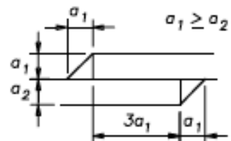
12) Ricoprimento semplice
