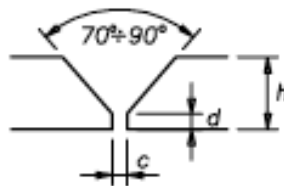
4) Bordi a V per h = 10 + 20 \text{ mm} c = 2 \text{ mm}; d = 3 \text{ mm} d=0 per h = 3 + 10 \text{ mm} d=3 per h = 11 + 20 \text{ mm} , necessaria ripresa al rovescio
