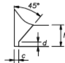
9) Preparazione a mezzo V per h = 5 + 30 \text{ mm}
