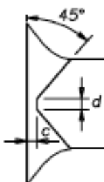
10) Preparazione a K per h = 10 + 30 \text{ mm}
