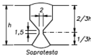
8) Giunto a doppio U per h = 30 + 50 \text{ mm} Consigliabile il tipo simmetrico se eseguito in piano
