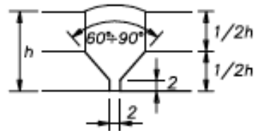
6) Preparazione a U per h = 20 + 30 \text{ mm} La ripresa a rovescio e' necessaria. Riduce il volume deposto
