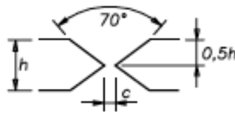
5) Bordi a X per h = 10 + 40 \text{ mm} c = 2 + 3 \text{ mm}
