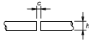
2) Bordi staccati verticali per h = 3 + 5 \text{ mm} c = h - 2 \text{ mm}
