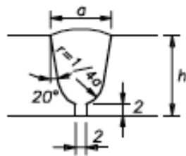
7) Preparazione a bicchiere per h = 20 + 30 \text{ mm} La ripresa e' necessaria. Riduce il volume deposto e facilita l'ingresso dell'elettrodo
