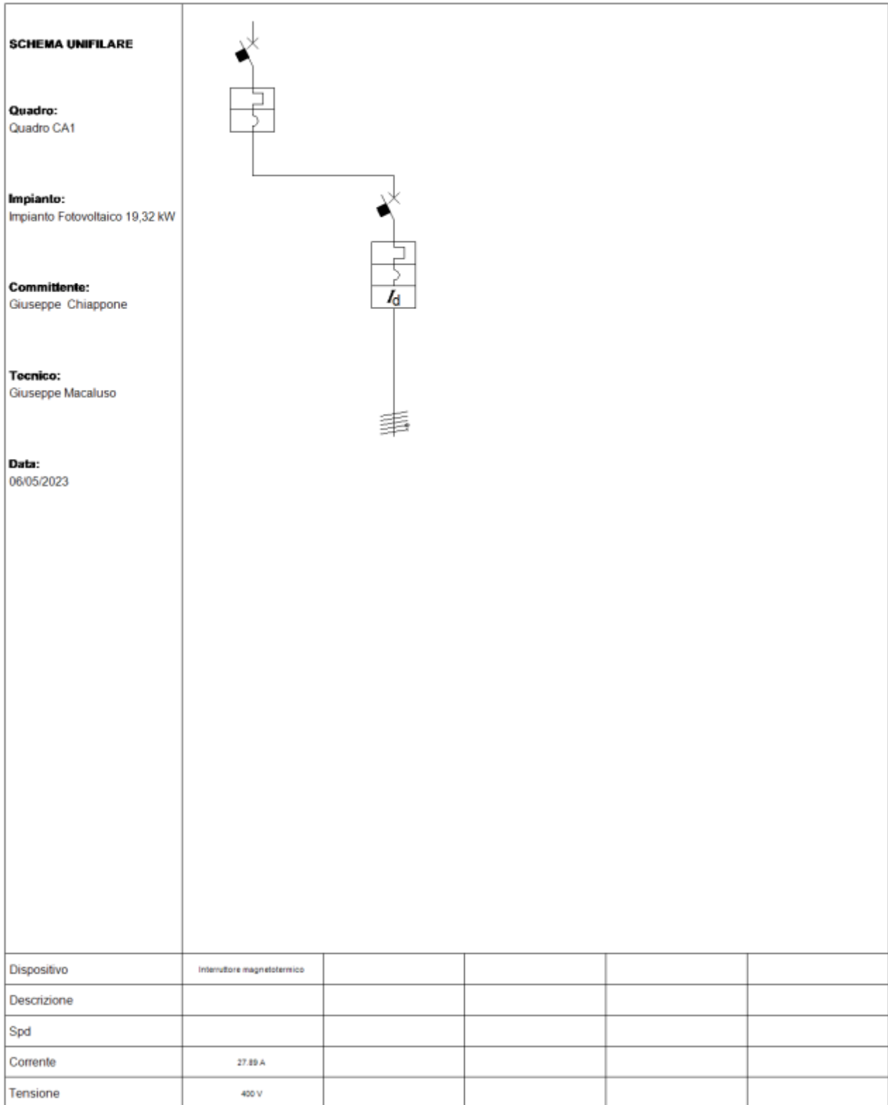
Fig. 7: Schema unifilare quadro "Quadro CA1"
