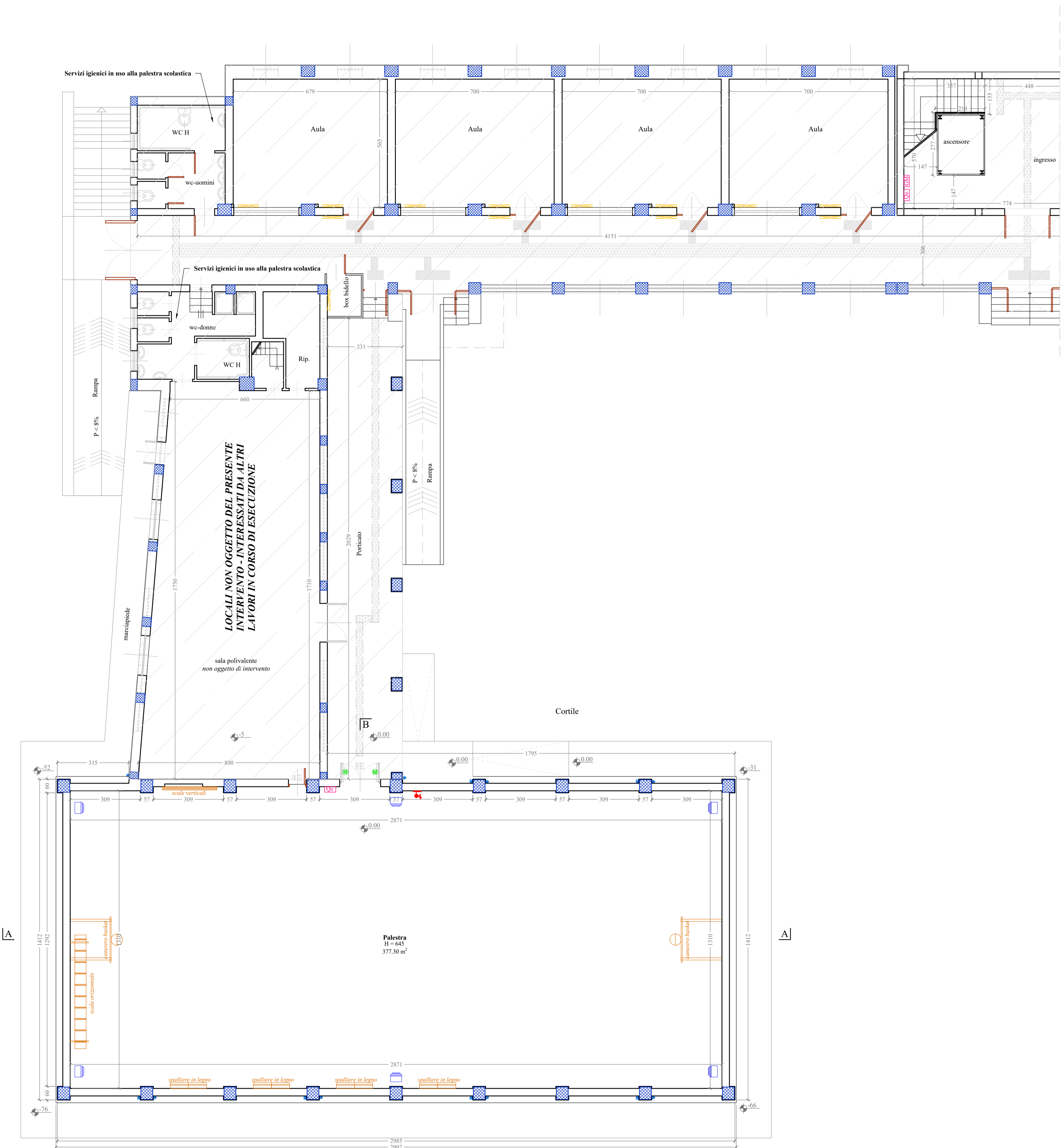
PIANTA PIANO TERRA
